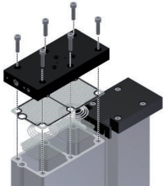
Plaat van de terugslagkleppen losmaken
