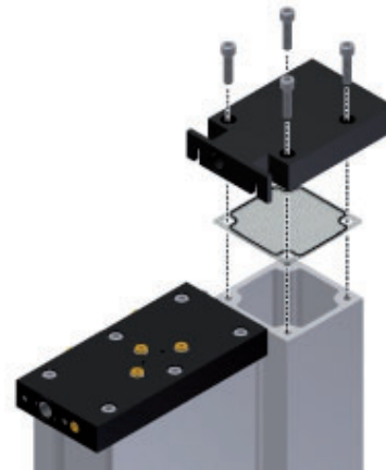
Kopplaat losmaken
