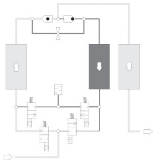
Opbouwen van druk
