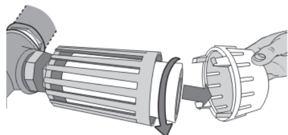
Geluiddemperelement vervangen
