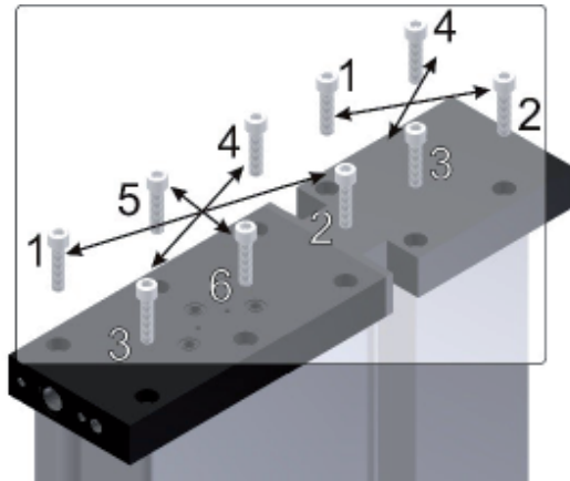
Terugslagventielplaat correct bevestigen
