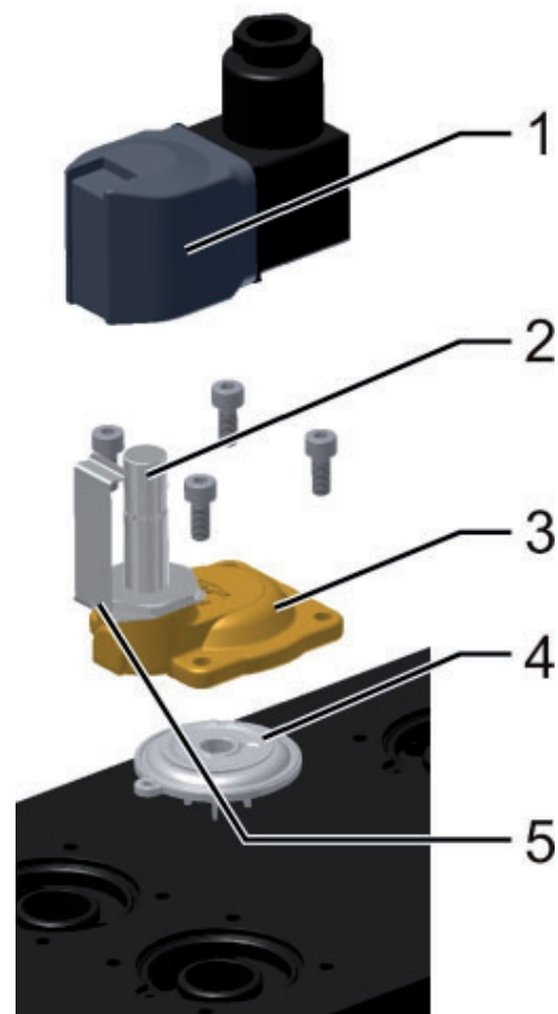
Magneetventiel
